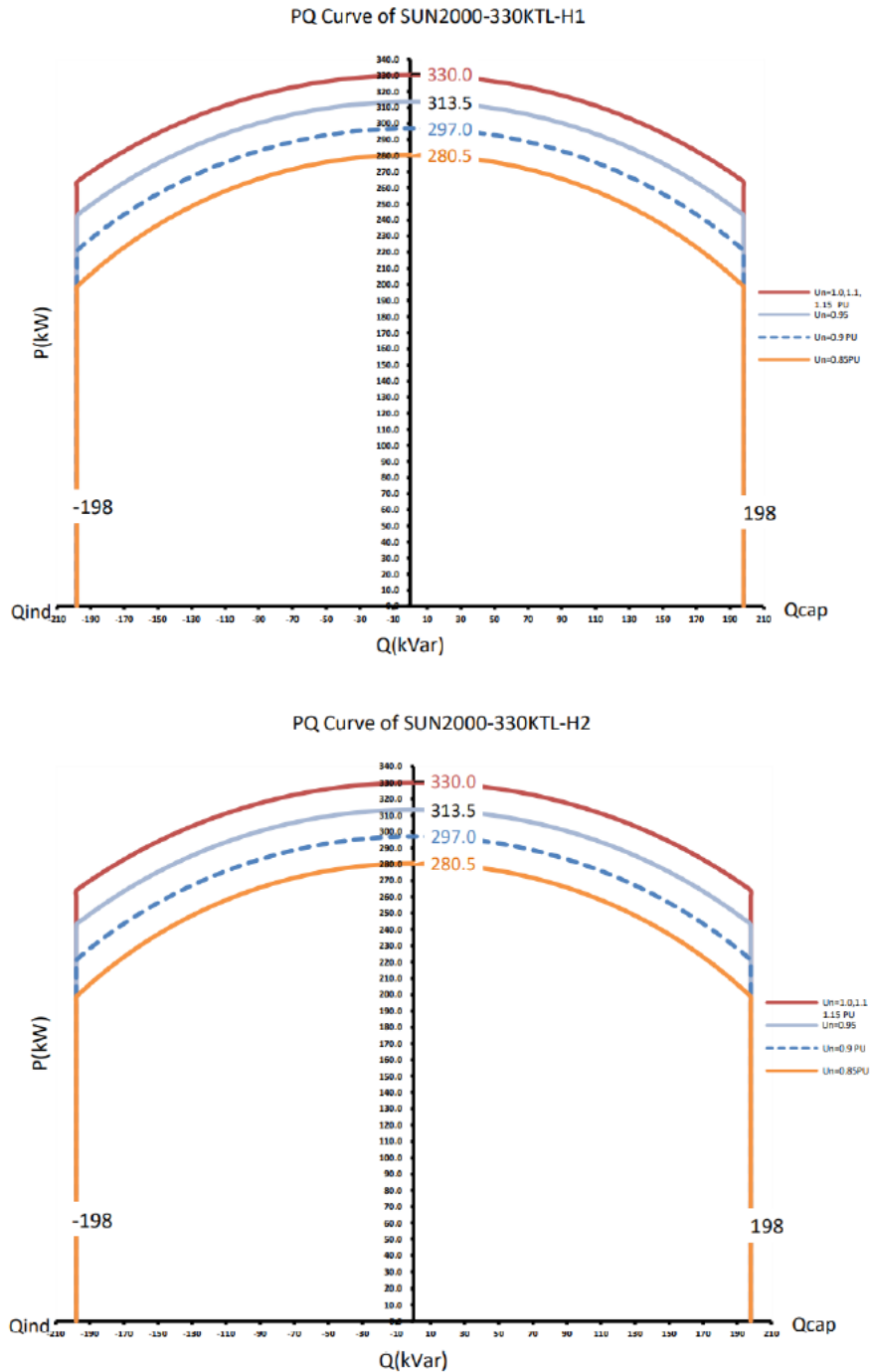
Abbildung 3: Blindleistungsstellbereich der SUN2000-330KTL-H1/H2, entnommen aus /1/
