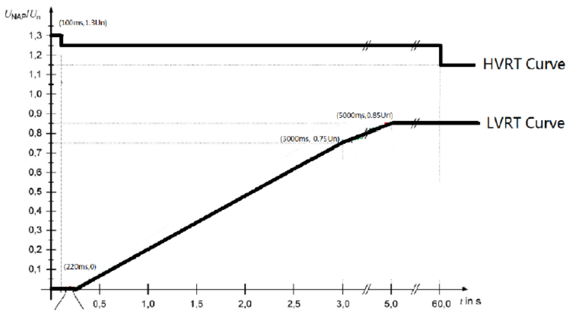
Abbildung 4: U(t)-Diagramm der SUN2000-330KTL-H1/H2, entnommen aus /1/
