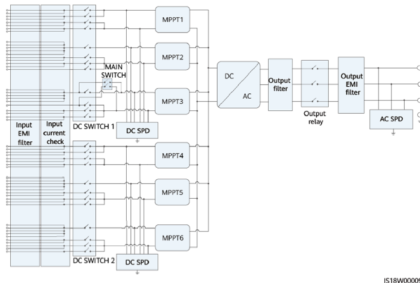
Abbildung 2: Schematische Übersicht der Erzeugungseinheit, entnommen aus /1/
