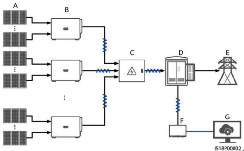
Abbildung 1: Schematische Übersicht des Anschlusses des Wechselrichters (B) an das Netz, entnommen aus /1/
