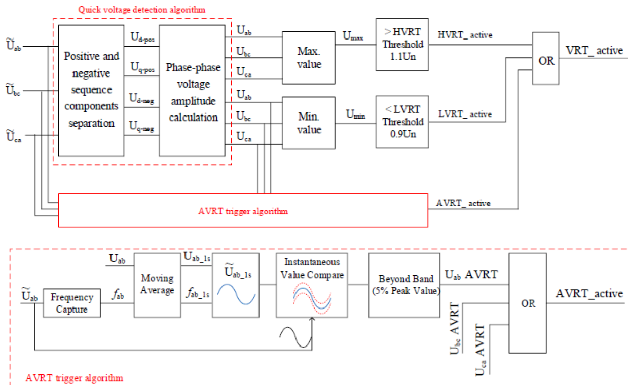
Abbildung 5: Die Implementierung der drei verschiedenen Fehlerauslöser (genannt HVRT, LVRT und AVRT) des SUN2000-330KTL-H1/H2. Die untere Abbildung ist eine einphasige Darstellung, aber die Funktion wurde für alle drei Phasen implementiert. /1/
